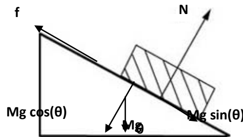
شکل ۲ - جسم روی سطح شیب دار
