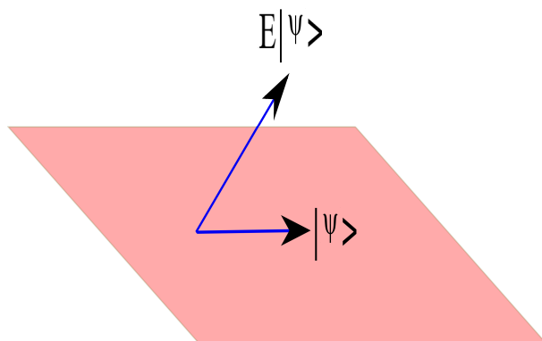
شکل ۸: خطاهای قابل شناسایی آنهایی هستند که حالت را از فضای کد خارج می کنند و از خود نشانه باقی می گذارند.
