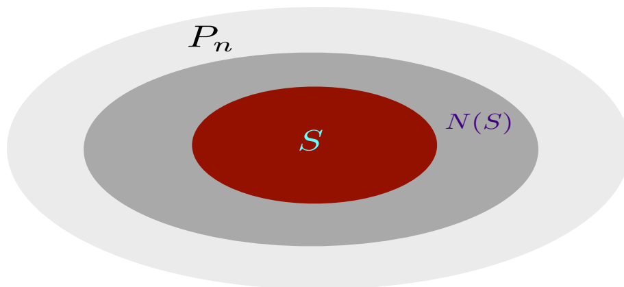
شکل ۵: گروه پاوولی، زیرگروه پایدارساز و گروه بهنجارساز این زیرگروه
