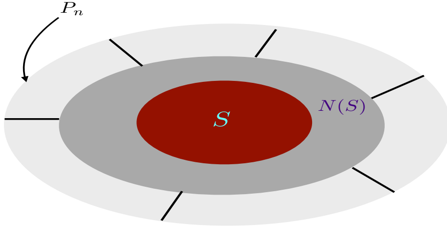
شکل ۷: گروه پاوولی، زیرگروه پایدارساز و گروه بهنجارساز این زیرگروه
