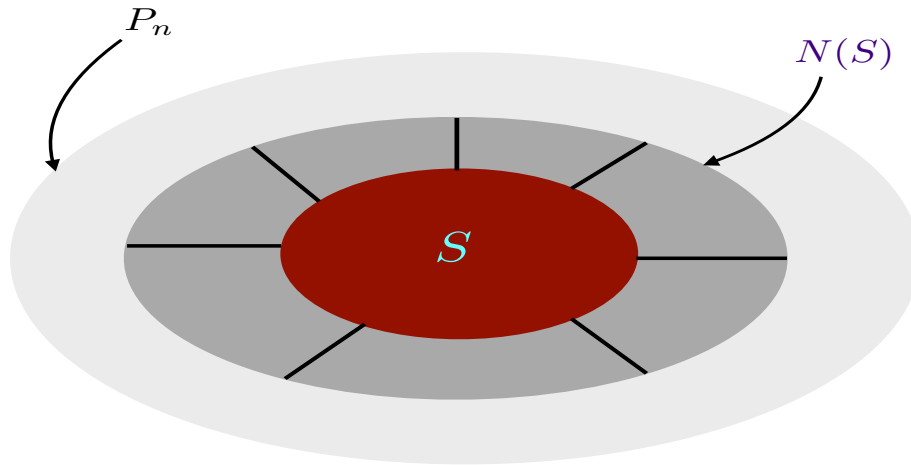
شکل ۶: گروه پاوولی، زیرگروه پایدارساز و گروه بهنجارساز این زیرگروه
